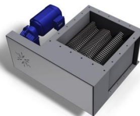
Klumpkross är den optimala lösningen för att krossa klumpar av t ex salt eller talk som har uppstått under hantering av materialet och som är tillräckligt mjuka för att kunna krossas.
