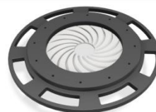
Irisspjäll (23) placeras under tömmarskålens utlopp. Kan enkelt strypa flödet och möjliggöra återknytning av säck.
