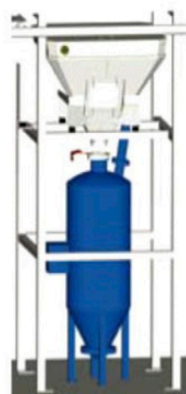
Trycksändare
