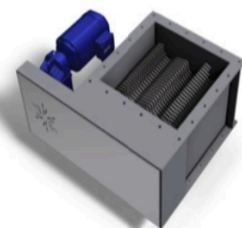
Klumpkross är den optimala lösningen för att krossa klumpar av t ex salt eller talk som har uppstått under hantering av materialet och som är tillräckligt mjuka för att kunna krossas.
