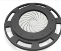
Irisspjäll (23) placeras under tömmarskålens utlopp. Kan enkelt strypa flödet och möjliggöra återknytning av säck.
