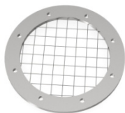
Galler (24). Placeras i botten av tömmarskålen för att hindra att operatör kan nå efterrustning (t ex skruv).
